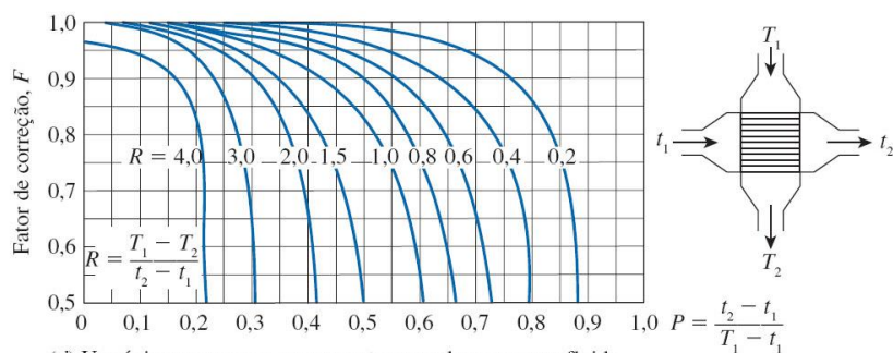
(d) Um único passe com escoamento cruzado e com um fluido com mistura e outro fluido sem mistura
