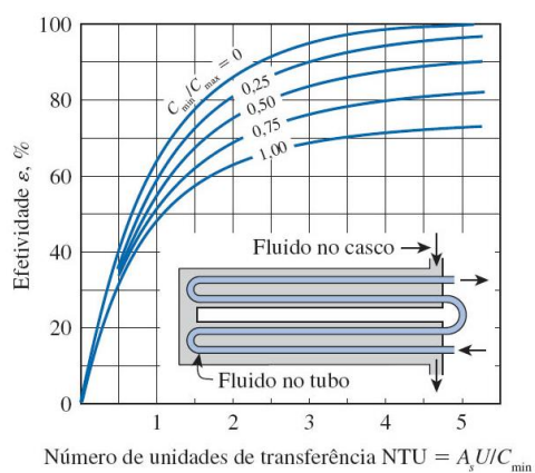
(d) Dois passes no casco e 4, 8, 12 (...) passes nos tubos
