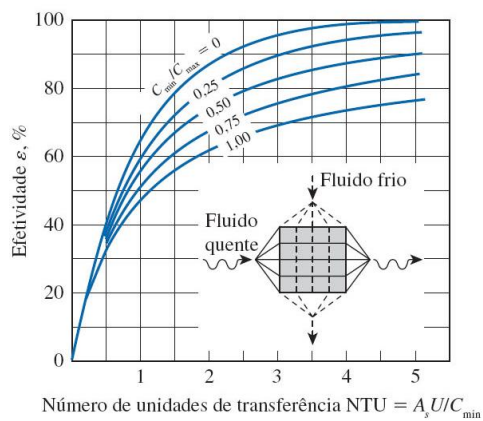
(e) Escoamento cruzado com dois fluidos sem mistura
