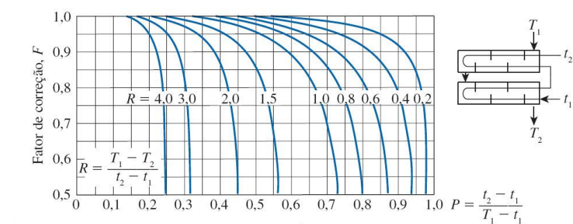
(b) Um passe no casco e 4, 8, 12, etc. (qualquer múltiplo de 4) passes nos tubos
