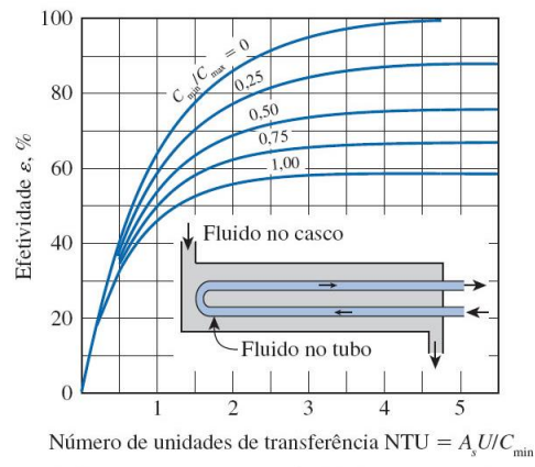
(c) Um passe no casco e 2, 4, 6 (...) passes nos tubos
