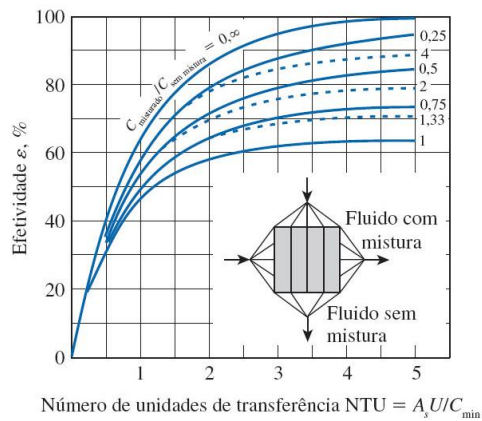
(f) Escoamento cruzado com um fluido com mistura e outro sem mistura
