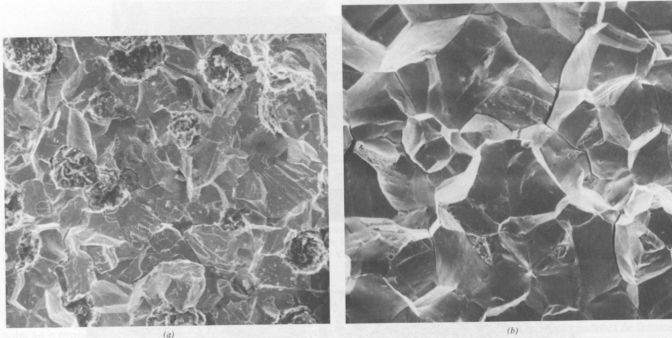
Fig. 8.6 (a) Fractografia eletrônica de varredura de ferro fundido dútil mostrando uma superfície de fratura transgranular. Ampliação desconhecida. (De V. J. Colangelo e F. A. Heiser, Analysis of Metallurgical Failures , 2nd edition. Copyright © 1987 de John Wiley & Sons, New York. Reimpresso sob permissão de John Wiley & Sons, Inc.) (b) Fractografia eletrônica de varredura mostrando uma superfície de fratura intergranular. 50×. (Reproduzido com permissão de ASM Handbook , Vol. 12, Fractography , ASM International, Materials Park, OH, 1987.)
