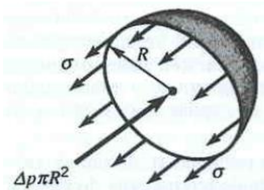
Diagrama de corpo livre da gota
