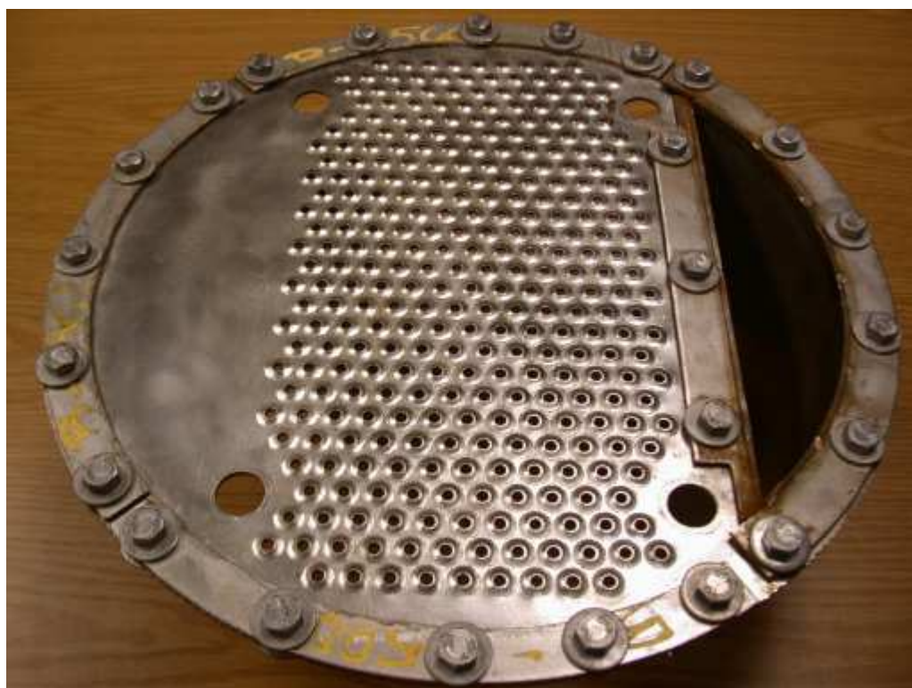
Prato com borbulhadores e transbordo
