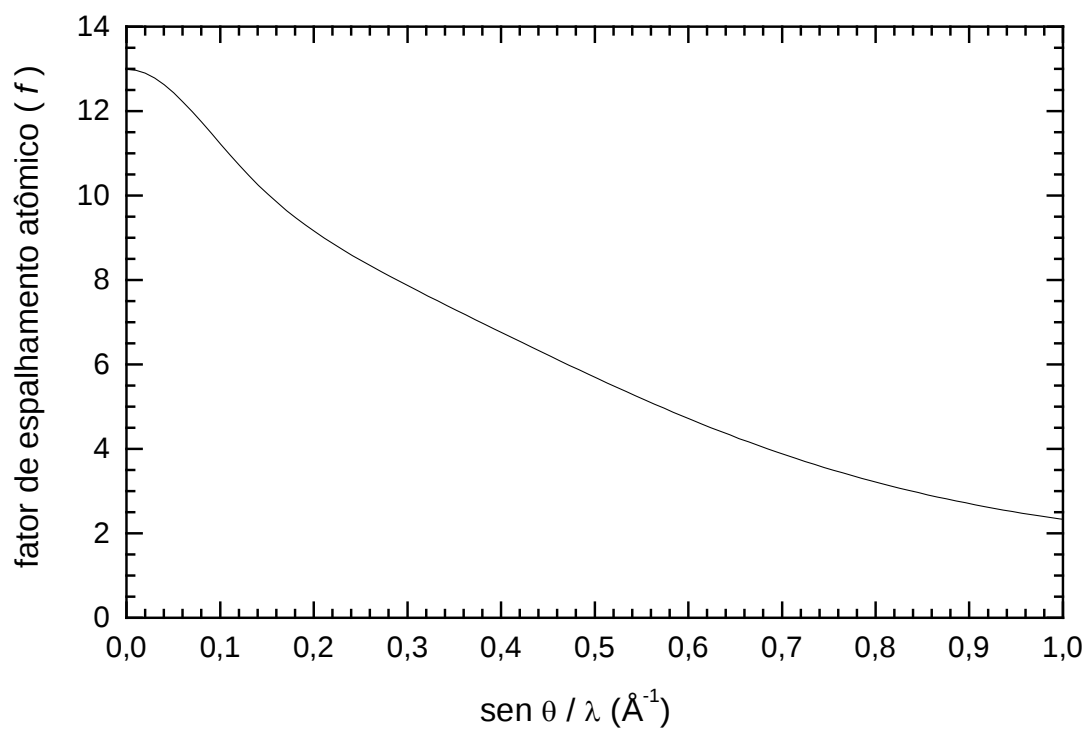
Fator de espalhamento atômico do alumínio
