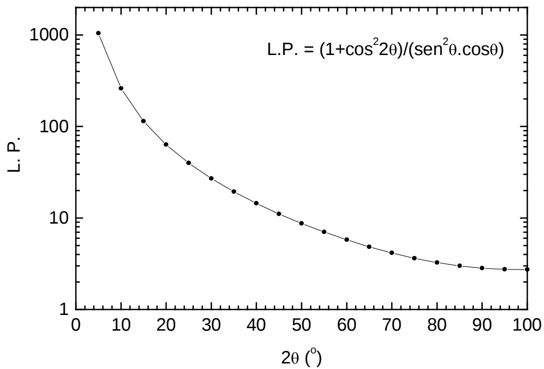
Fator de Lorentz - Polarização
