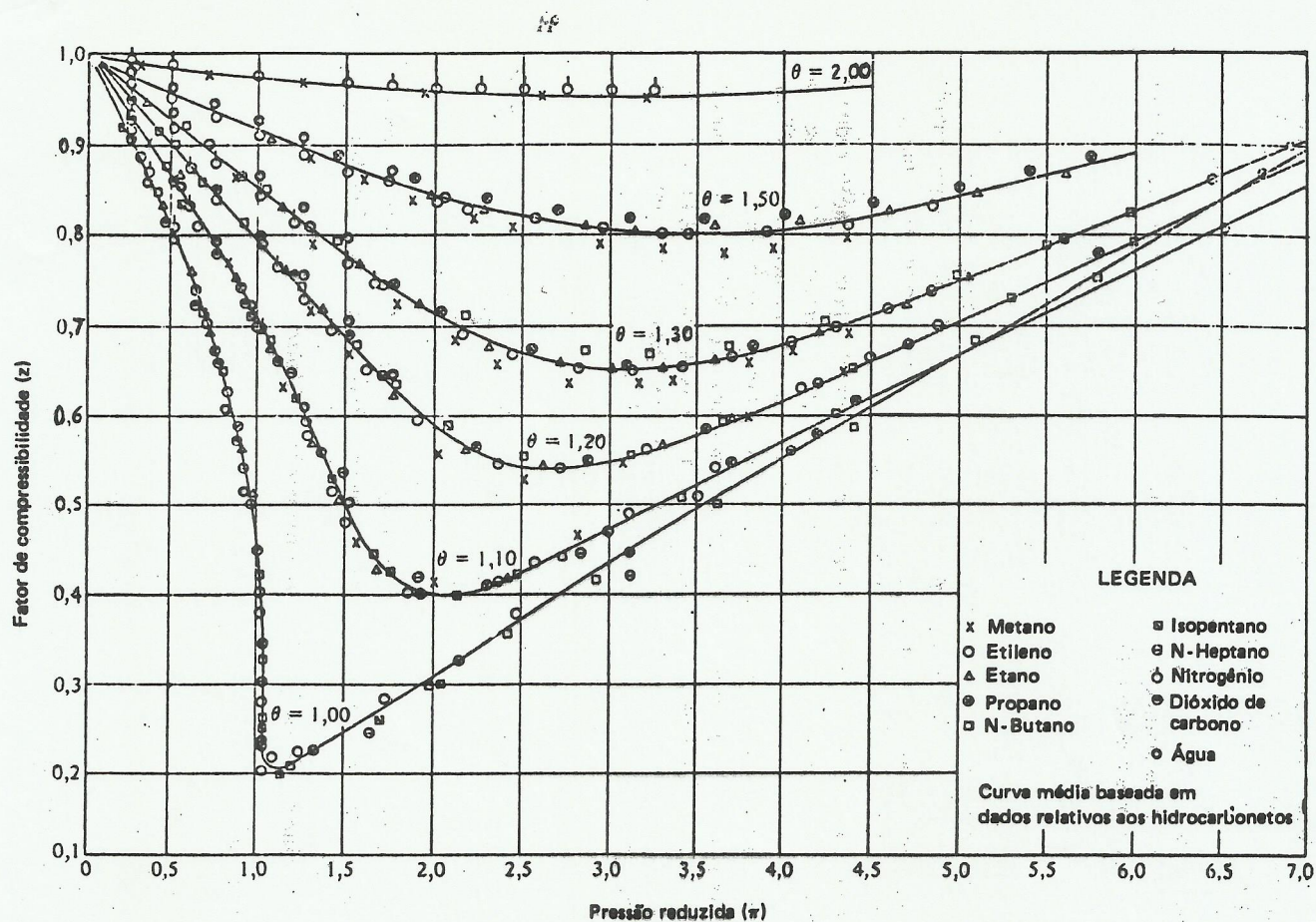
Fig. 3.15. Verificação da Lei dos Estados Correspondentes (Gouq-Jen Su, 1946).
