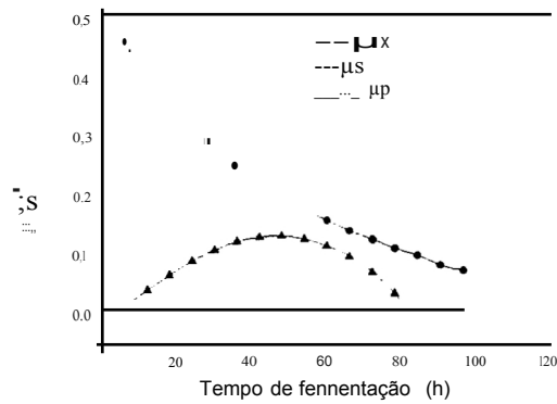
FIGURA 22: Velocidades específicas do experimento 3 (vazão de ar de 60 ml/min e fator de concentração de hidrolisado de 3,50 vezes).
