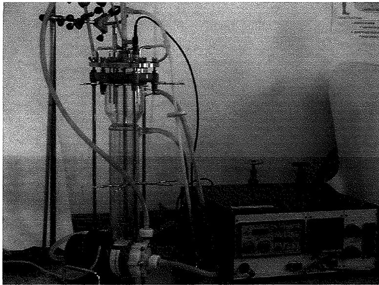
FIGURA 2: Biorreator de coluna de bolhas utilizado no presente trabalho.
