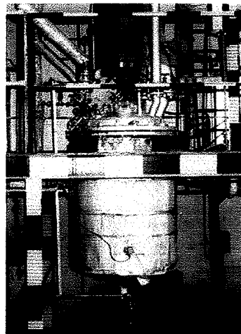
FIGURA10: Reator de hidrólise do bagaço de cana (250 litros) utilizado no presente trabalho.
